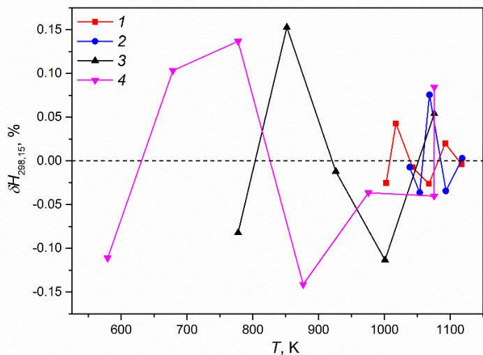
Рисунок 4 – Относительные отклонения измеренных значений энтальпии жидких сплавов Li–Pb от аппроксимационных уравнений.
