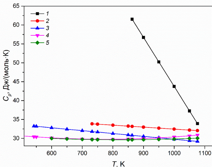
Рисунок 5 – Теплоемкость жидких сплавов К–Рб
