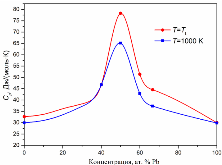
Рисунок 6 – Концентрационные зависимости теплоемкости жидких сплавов Cs–Pb при температуре ликвидуса и 1000 К
