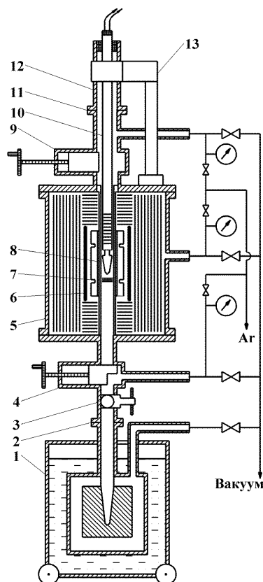
Рисунок 1 – Общая схема калориметра.
