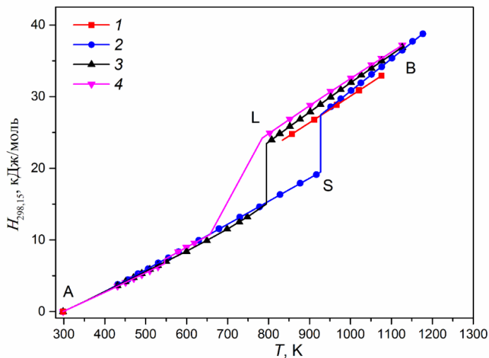
Рисунок 3 – Измеренные значения инкремента молярной энтальпии сплавов Cs–Bi в твердом (AS) и жидком (LB) состояниях.
