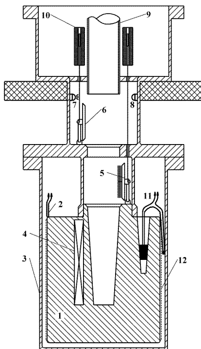
Рисунок 2 – Калориметрический узел.
